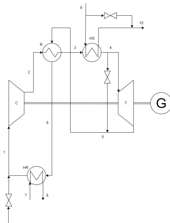
Rysunek 1. Punkty pomiarowe układu
